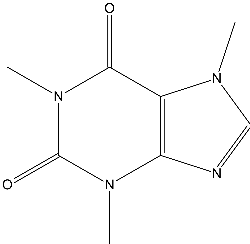
Caffeine
